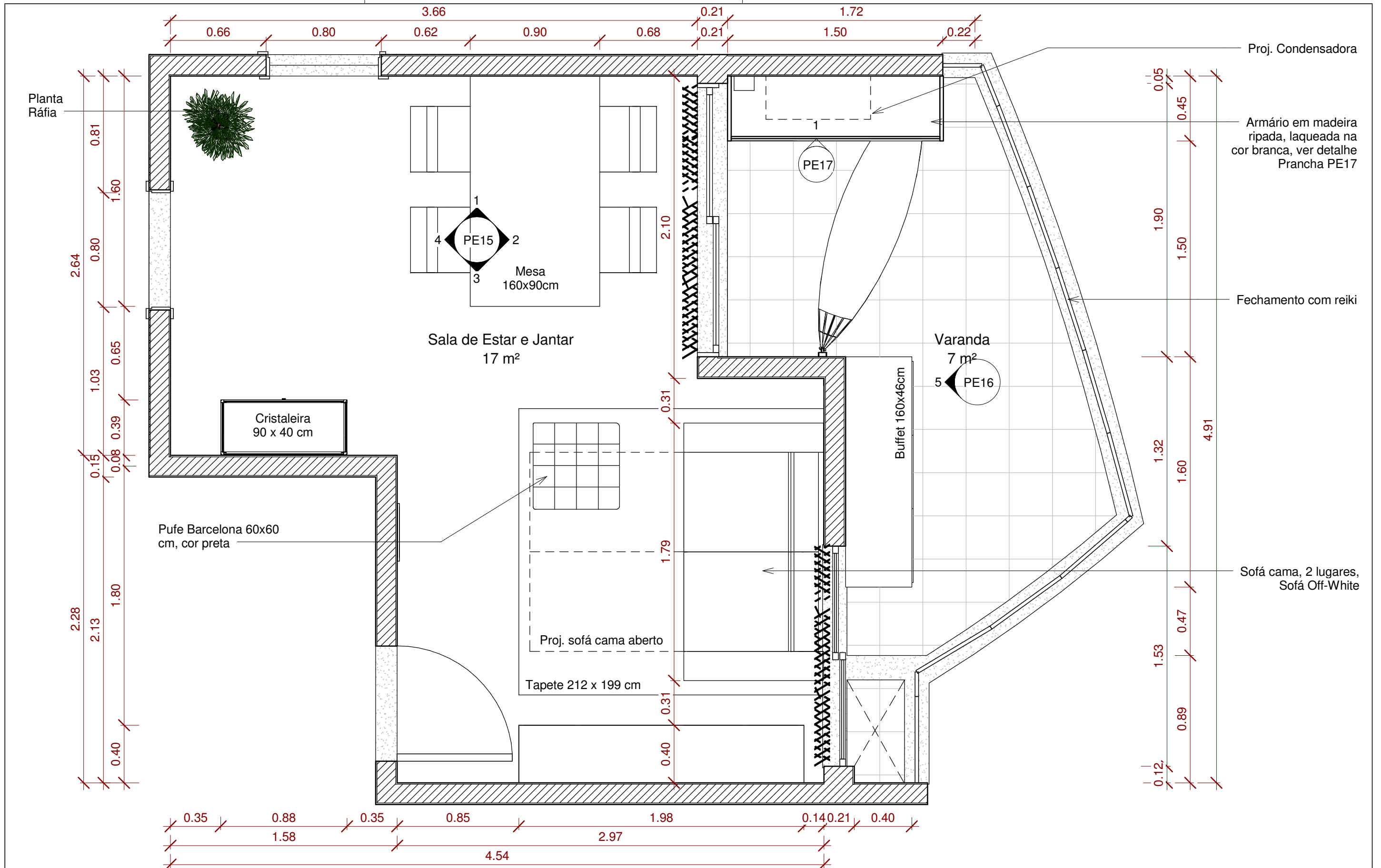
1 Planta Baixa - Sala Estar/Jantar e Varanda 1 : 25
