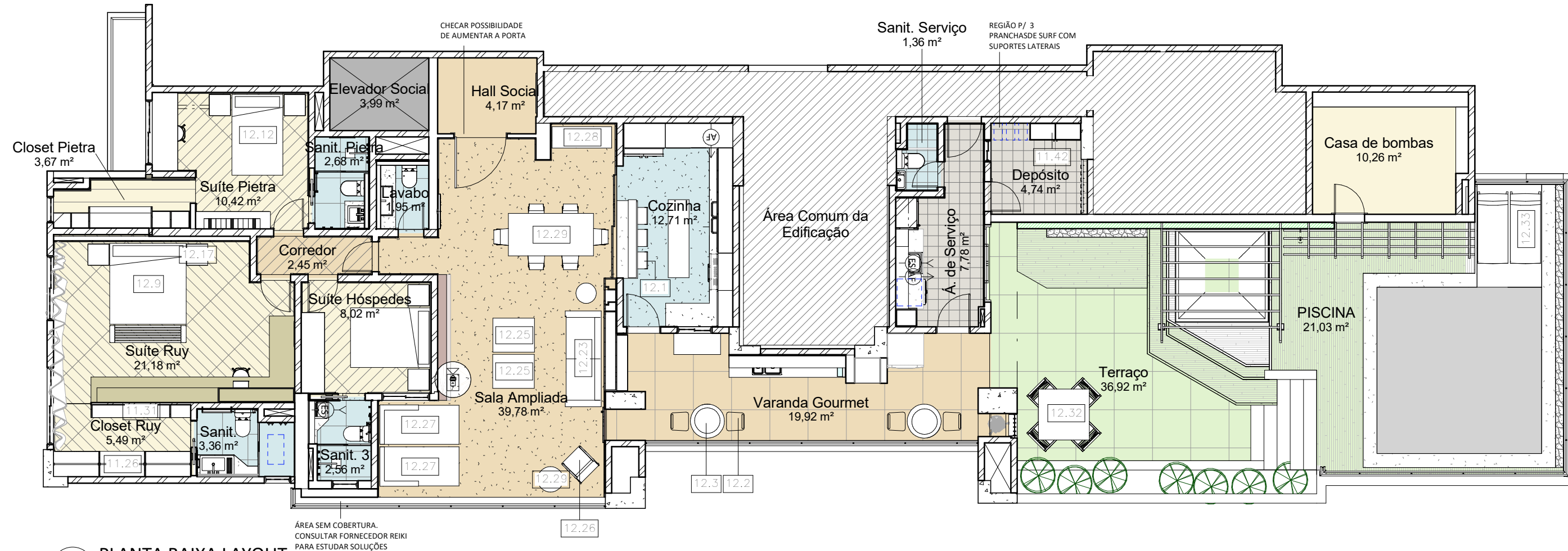
1 PLANTA BAIXA LAYOUT ESCALA 1:100
