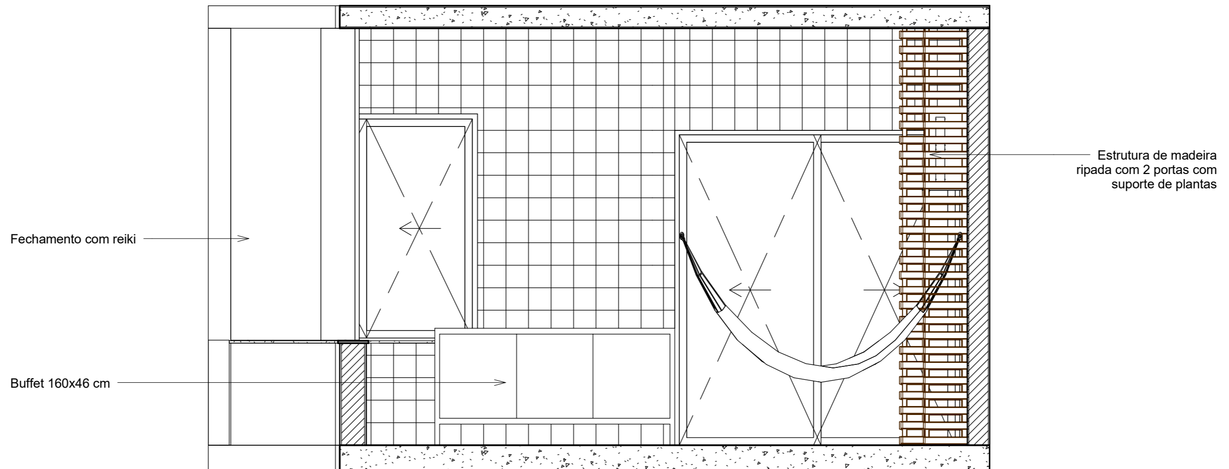
1 Vista 5 - Varanda 1 : 25
