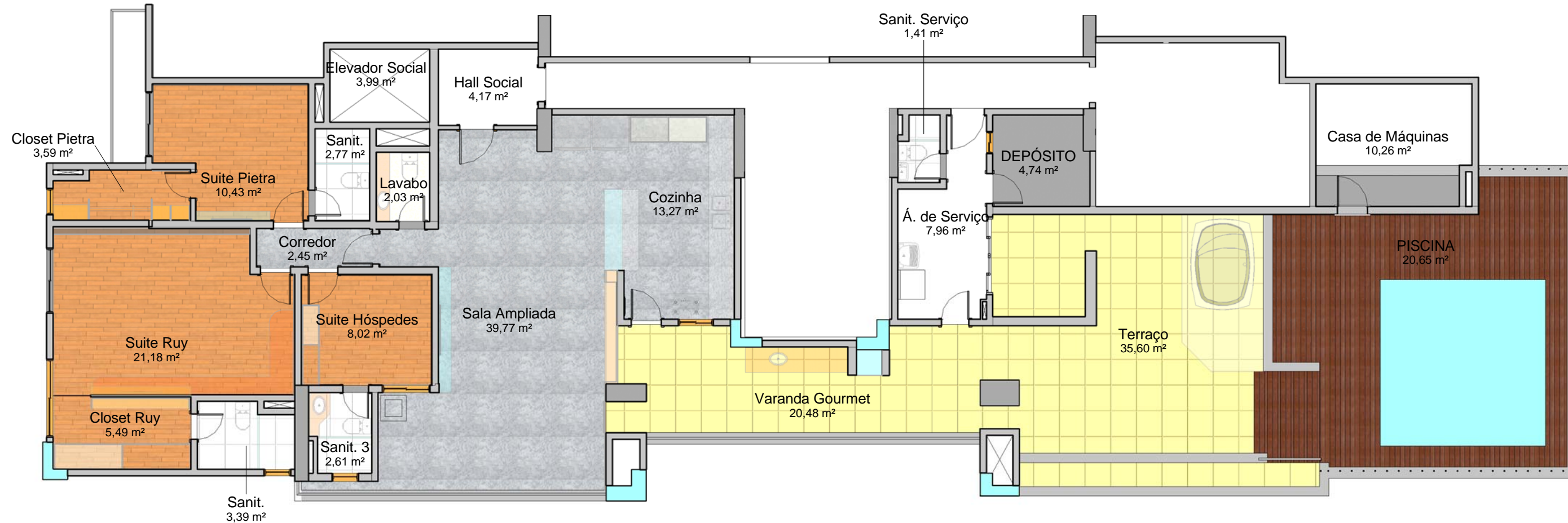
1 PLANTA BAIXA LAYOUT ESCALA 1 : 100
