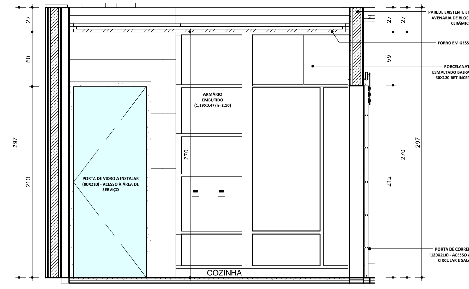
5 COZINHA - VISTA D ESCALA 1:25
