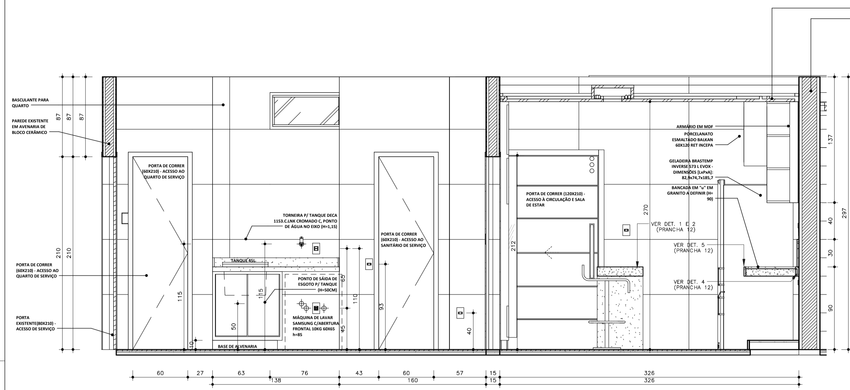
2 COZINHA - VISTA A ESCALA 1:25
