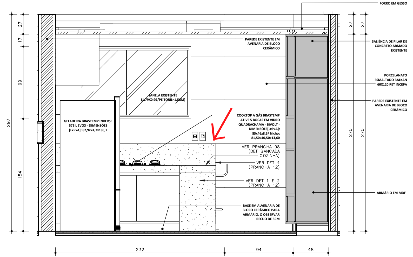
4 COZINHA - VISTA C ESCALA 1:25
