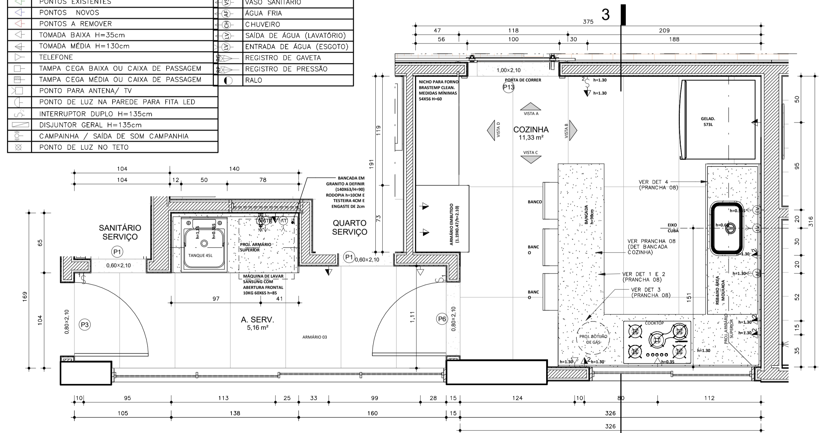
1 PB COZINHA E A.SERV. ESCALA 1:25
