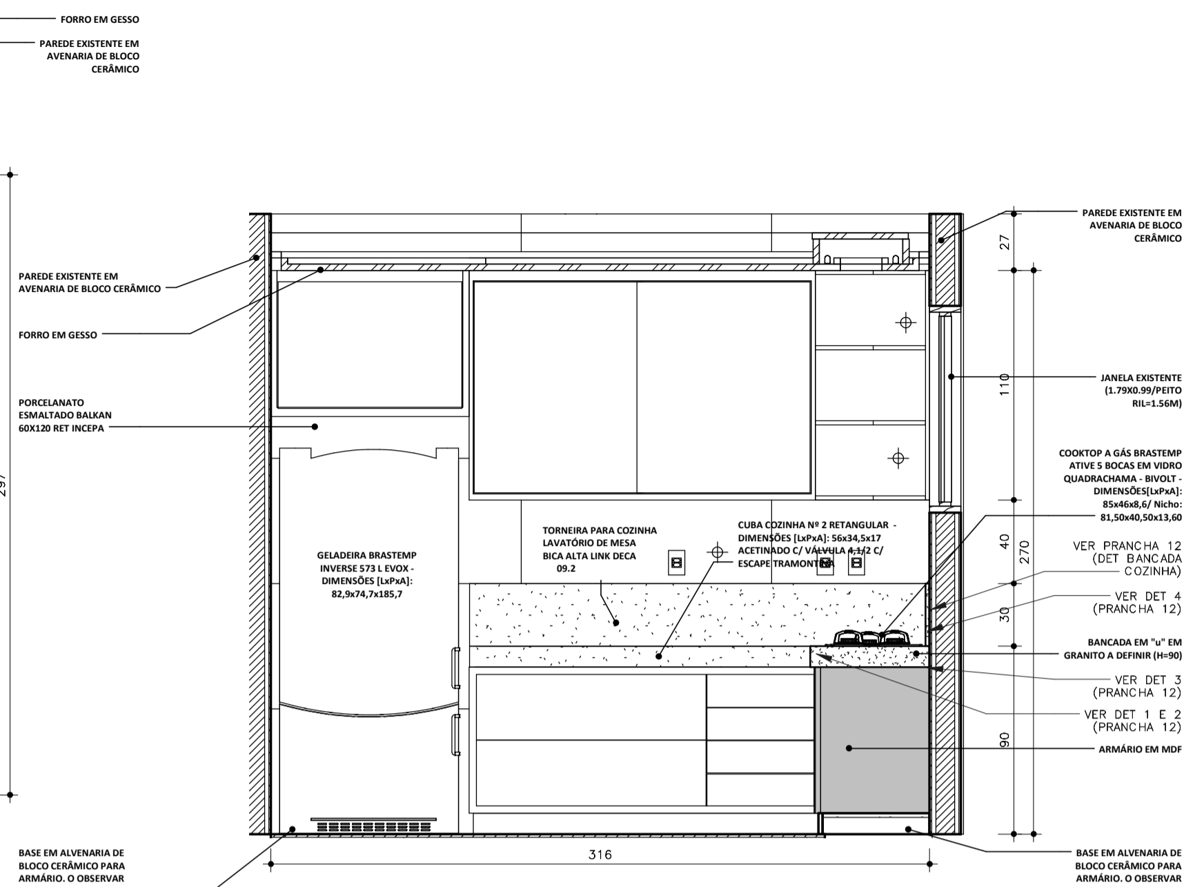
3 COZINHA - VISTA B ESCALA 1:25
