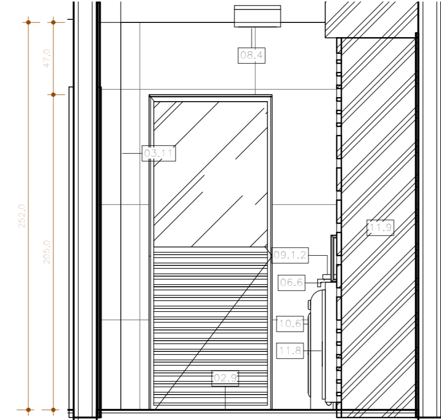
5 ÁREA DE SERV. - VISTA D ESCALA 1:25
