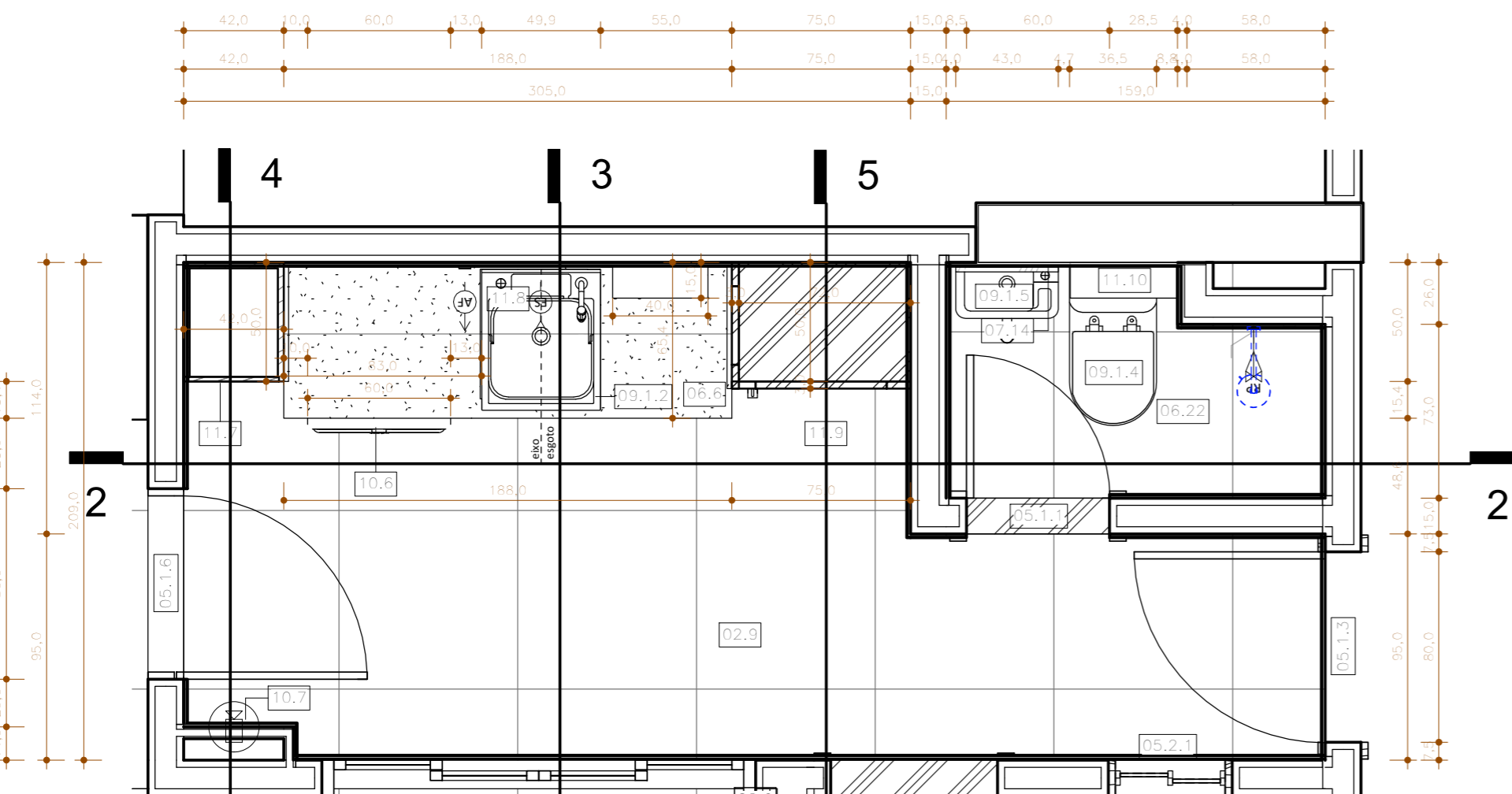
1 PB ÁREA DE SERVIÇO ESCALA 1:25
